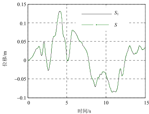
图 7 节点 S 与 S 1 位移比较
