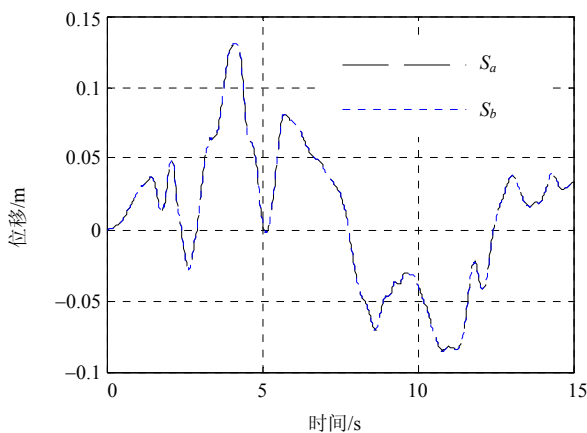
图 12 节点 S_a 与 S_b 位移比较
