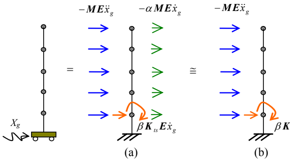
图 1 位移输入模型等效分解示意图
